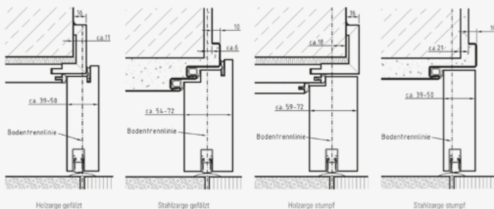
Unterschiedliche Ausführungsvarianten der Bodenschwelle
