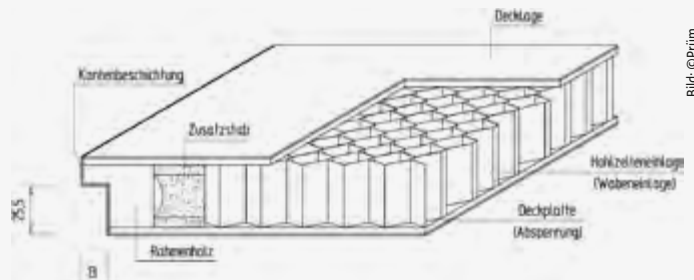
Innenleben einer Wabentür
