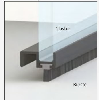
Eine Bürste schließt die Tür zum Boden ab.
