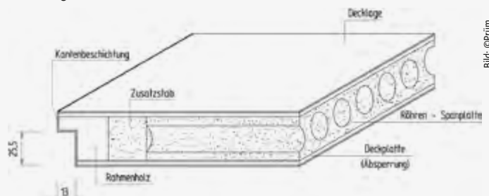
Innenleben einer Röhrenspantür
