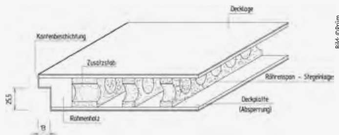
Innenleben einer Röhrenspanstreiftür
