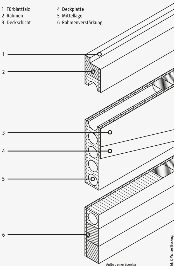
Aufbau einer Sperrtür
