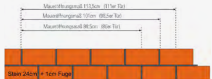
Baurichtmaße als Maßketten in der Breite
