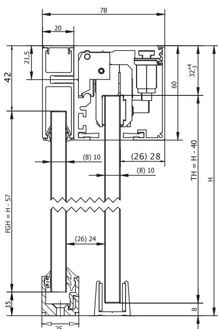
Motion 1300 – Querschnitt Deckenbefestigung mit Festteil
