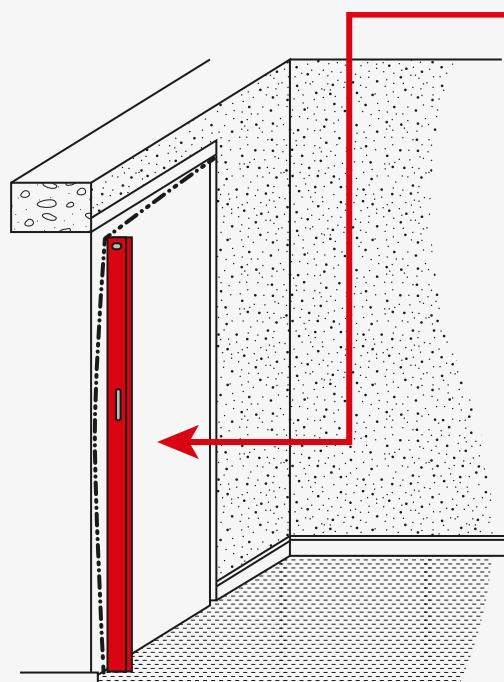
Bestimmung der Durchbiegung an einem Türblatt
